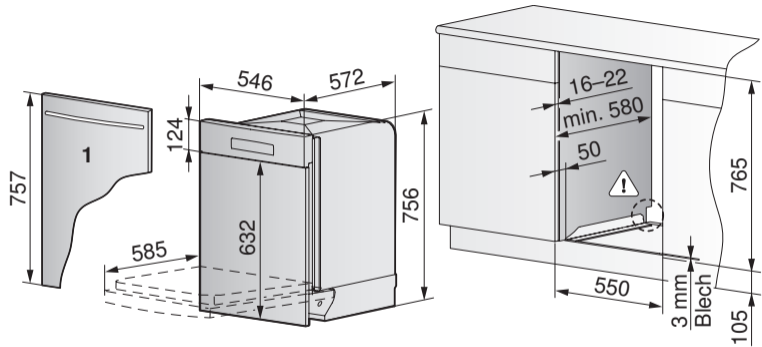
Lave-vaisselle GS 55 Swiss Premium Line, Norme SMS / largeur de la niche 55 cm
